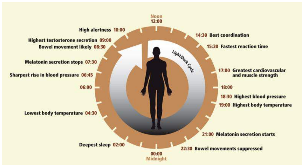
Figuur 5: het gemiddelde 24-uurs ritme van ons lichaam. Tijden zijn gebaseerd op de eigen lokale zonnetijd (zie deel 2a), pieken en dalen gebaseerd op die van een gemiddeld dagmens . Afhankelijk van het persoonlijke chronotype kunnen deze pieken en dalen uren eerder of later plaatsvinden (zie deel 2e).
